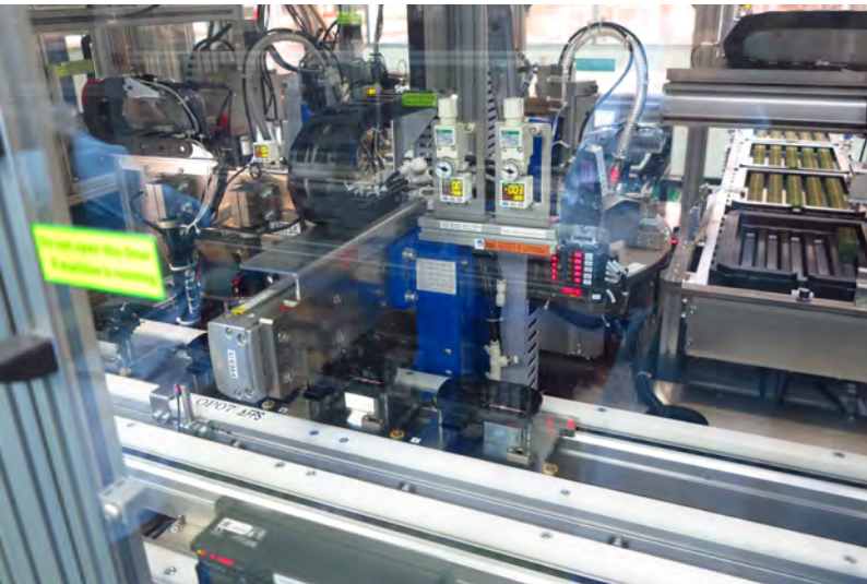
กระบวนการประกอบชุดย่อยตัวครอบเฟืองเกียร์
